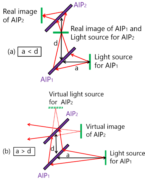
図 6 実像鏡の間隔による空中像の結像位置の違い
