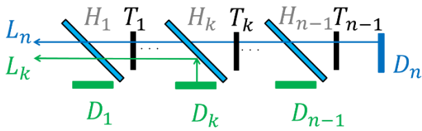
図 4 オクルージョン表現可能な N 層化
