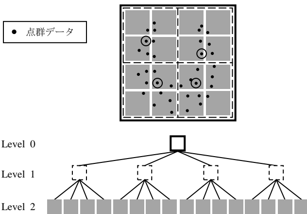
図4 完全4分木
