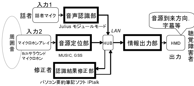
図 1: システムブロック図
